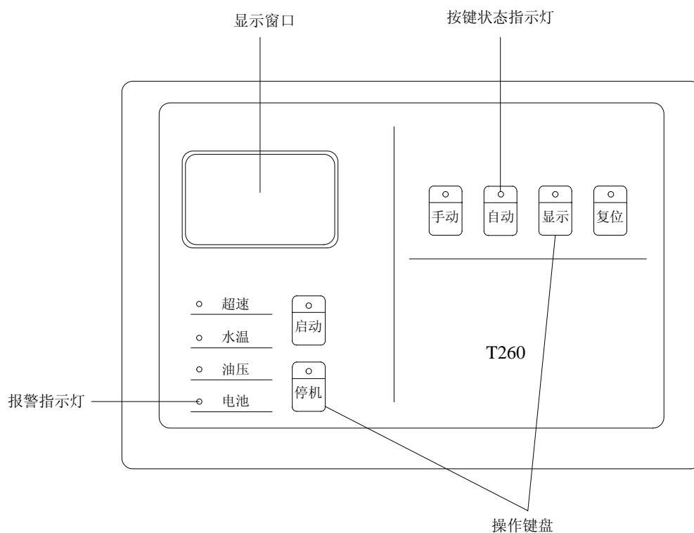
图 1-1. T260N 前面板
