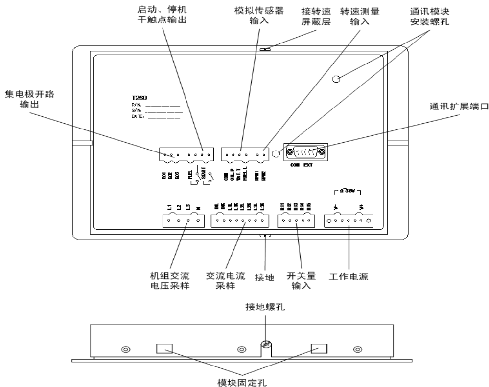
图 1-2. T260N 后面板
