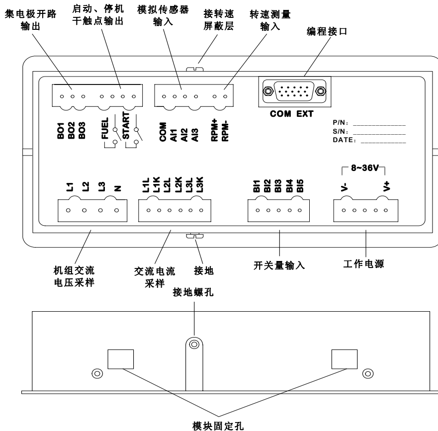
图 1-2 T210N 后面板
